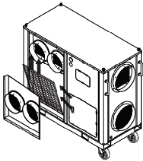
Рисунок 11 - извлечение фильтра
